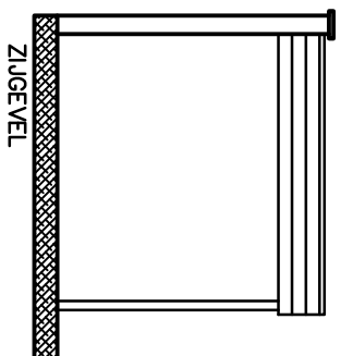
DOOSNEDE B
