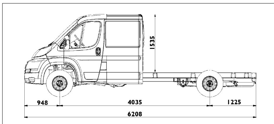
Lange wielbasis verlengd Empattement long rallongé
