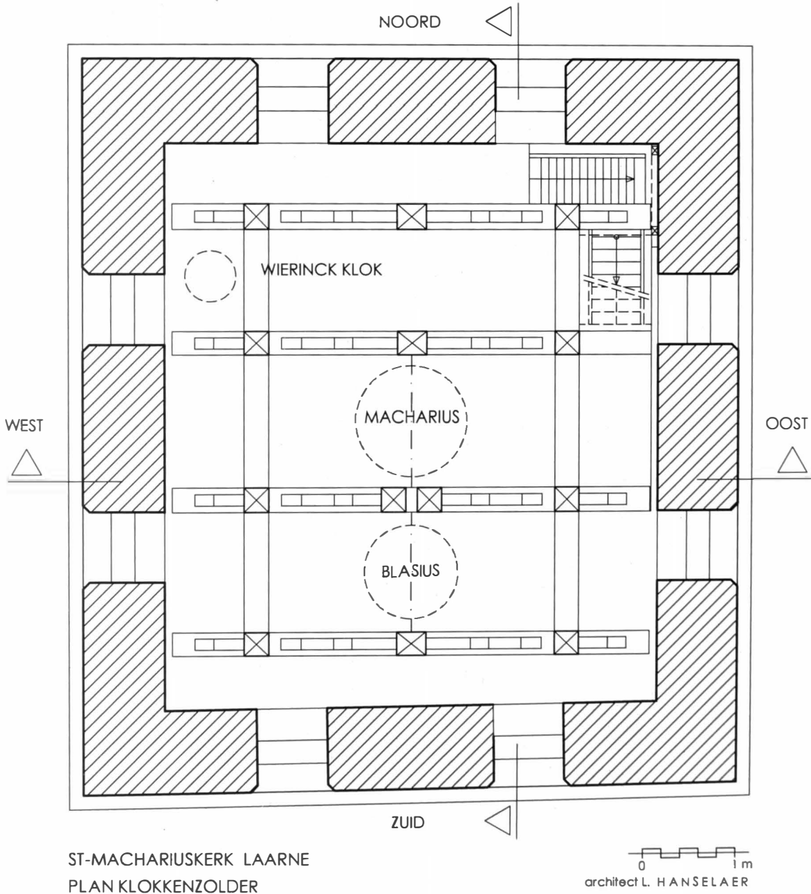
Illustratie 5. Sint-Machariuskerk Laarne. Plan van de klokkenzolder door architect Lieven Hanselaer, 2009.
