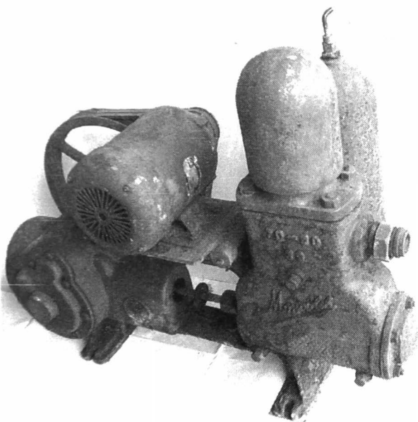
Fig. 4: Waterpomp voor grondwater.
