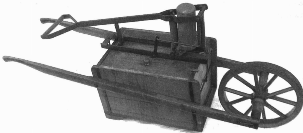
Fig. 7: Houten sproeikar voor besproeiing met een aftreksel van tabaksnerven.
