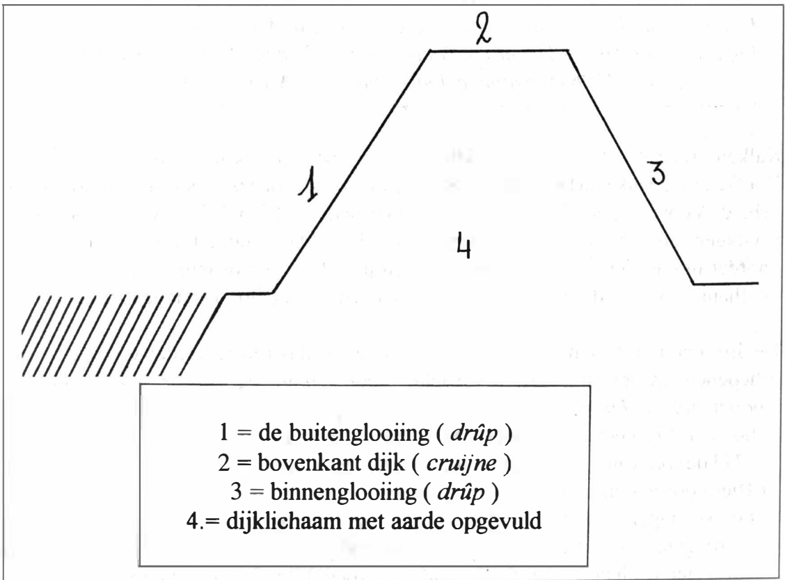
Figuur 3. Doorsnede van een dijk 24
