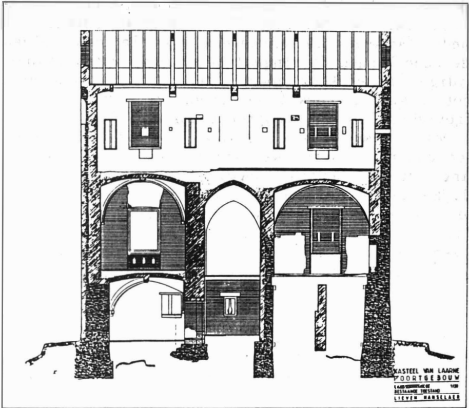
Fig. 3. : Langsdoorsnede over het poortgebouw, bestaande toestand.
