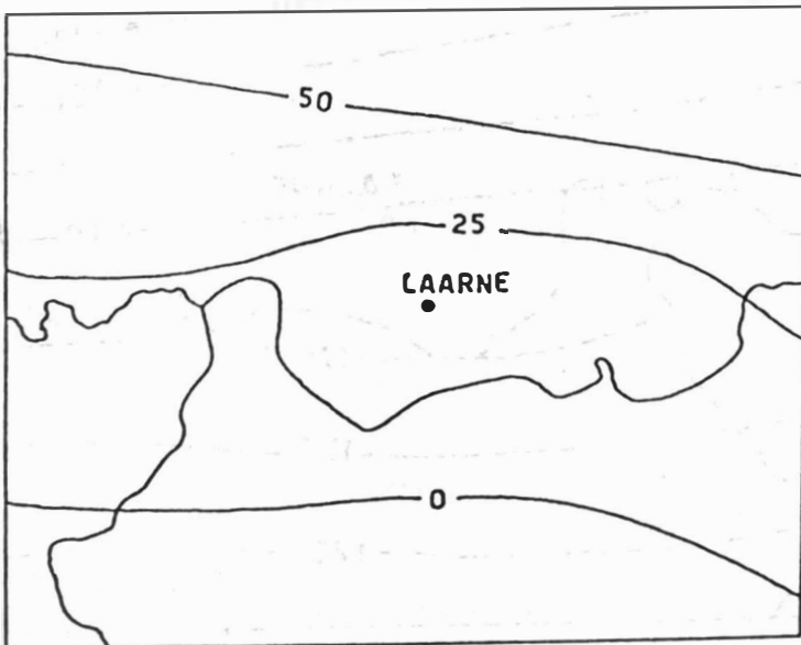
Fig. 4 : Dikte van het Krijt (naar Jacobs P., 1968).
