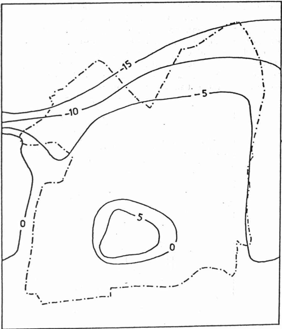
Fig. 6 : Isohypsens van de top van het Tertiair (naar Jacobs P., 1968).
