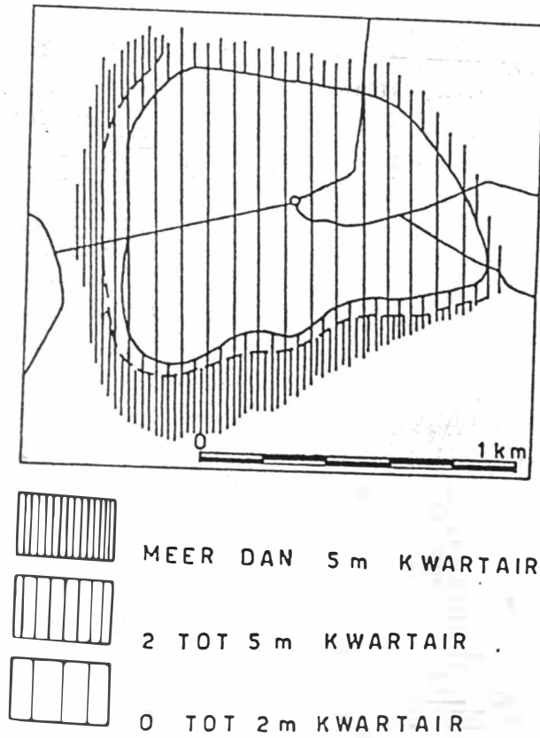
Fig. 8 : Dikte van het Kwartair te Laarne-dorp (naar Jacobs P., 1968).
