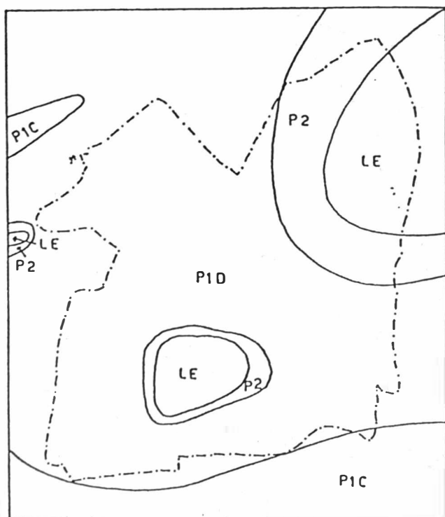
Fig. 5 : Geologische schetskaart van het Tertiair te Laarne (naar Jacobs P., 1968).
