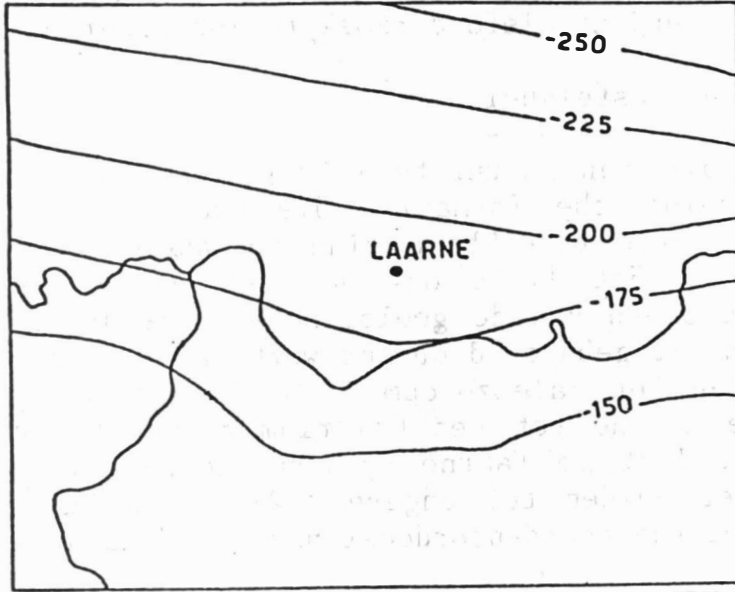
Fig 3. : Isohyspen van de top van het Krijt (naar Jacobs P., 1968).
