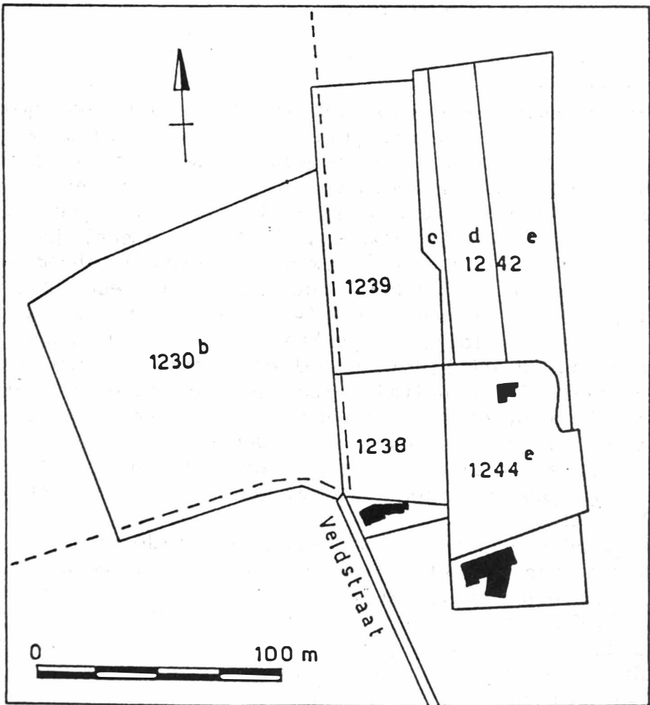
Fig. 10 : Lokalisatie van de steengroeve te Laarne-dorp (naar Balthau E., 1984).
