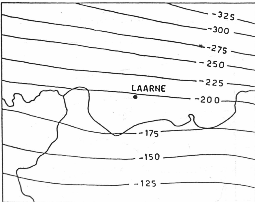
Fig. 2 : Isohypsen van de top van het Paleozoicum (naar Jacobs P., 1968).
