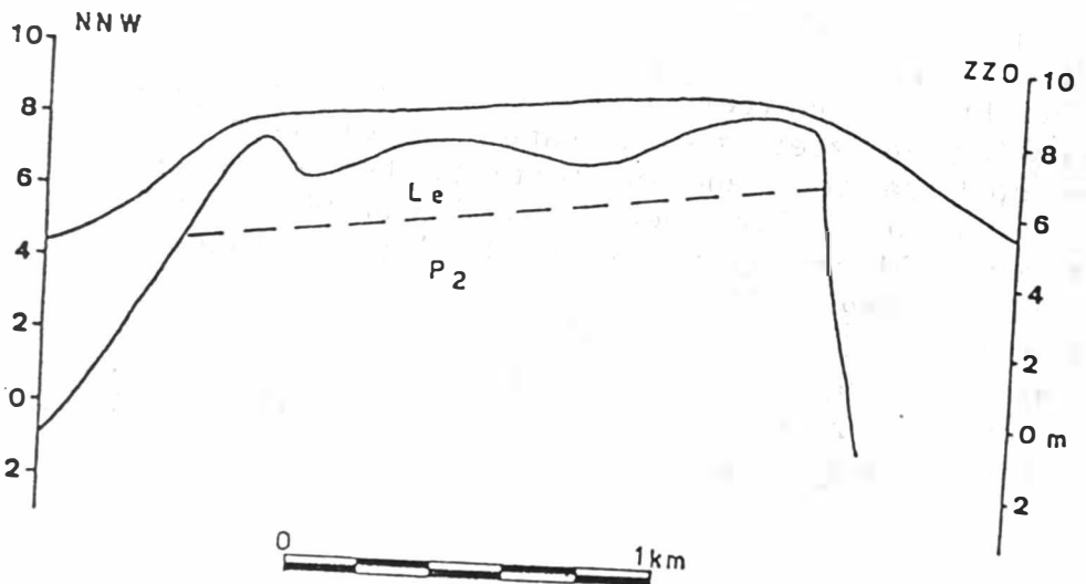
Fig. 8 : Dikte van het Kwartair te Laarne-dorp (naar Jacobs P., 1968).
